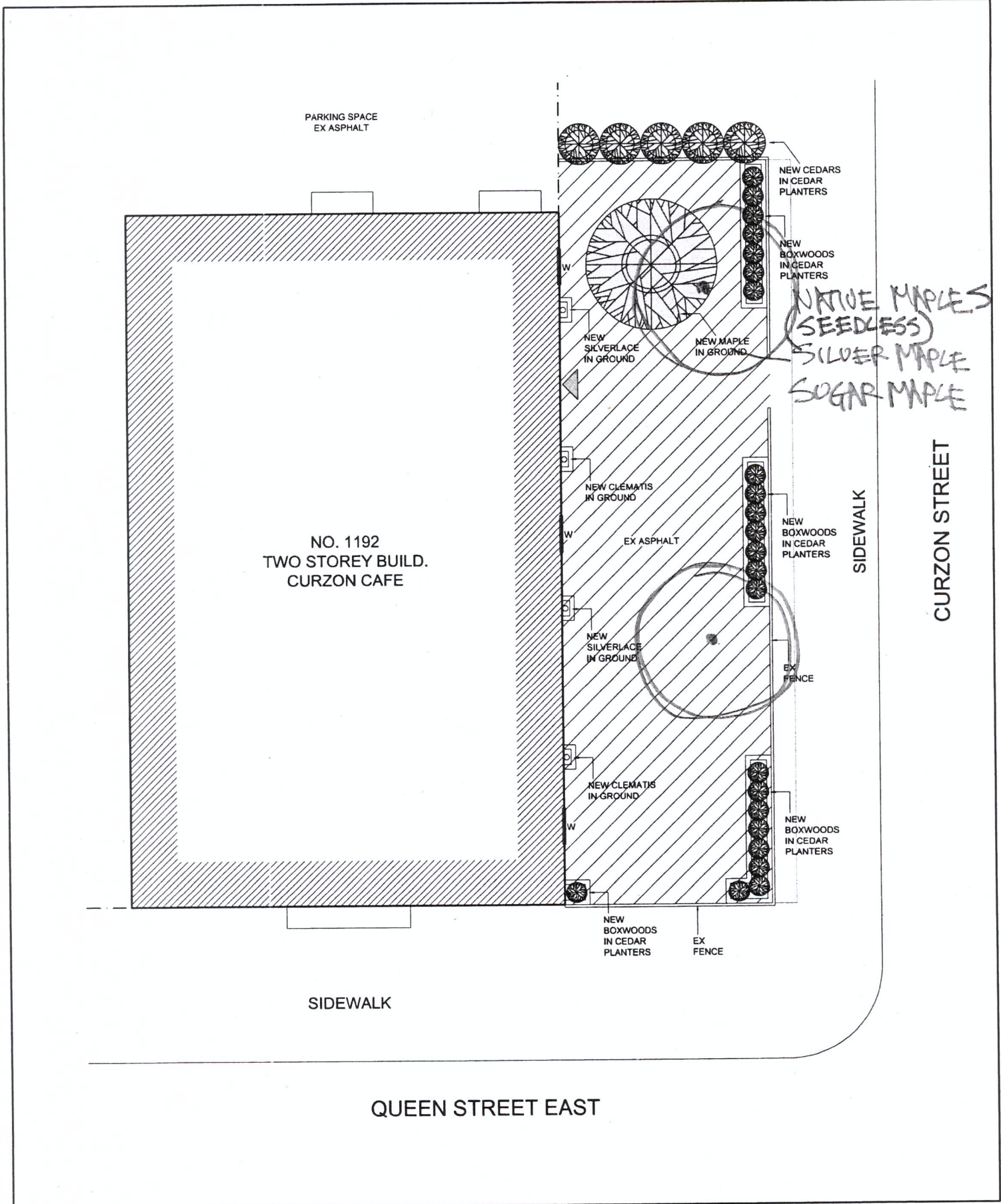
1192 CURZON ST. LANDSCAPE PLAN SCALE: 1/8" = 1'0"
