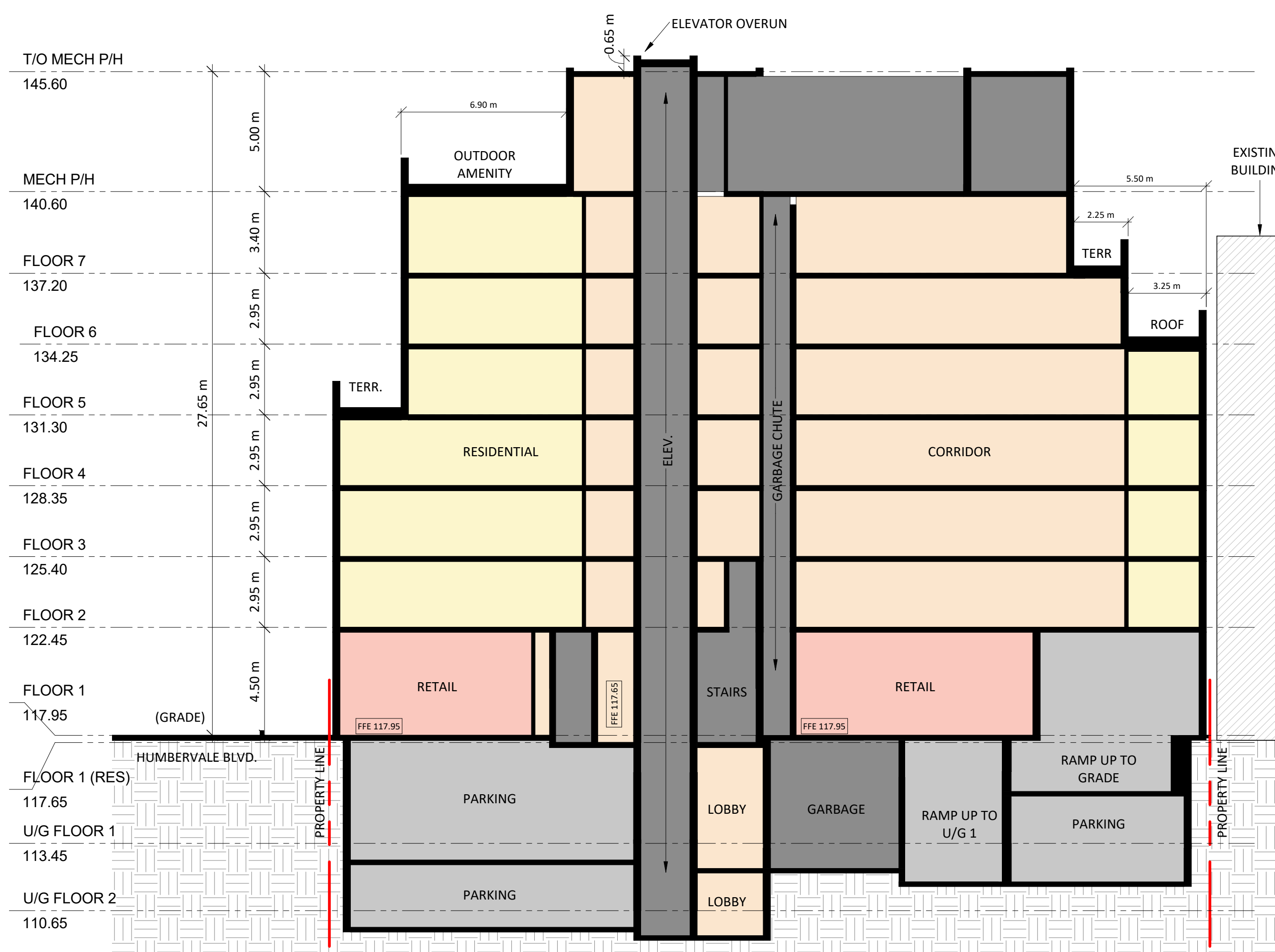
D SECTION D 1 : 150
