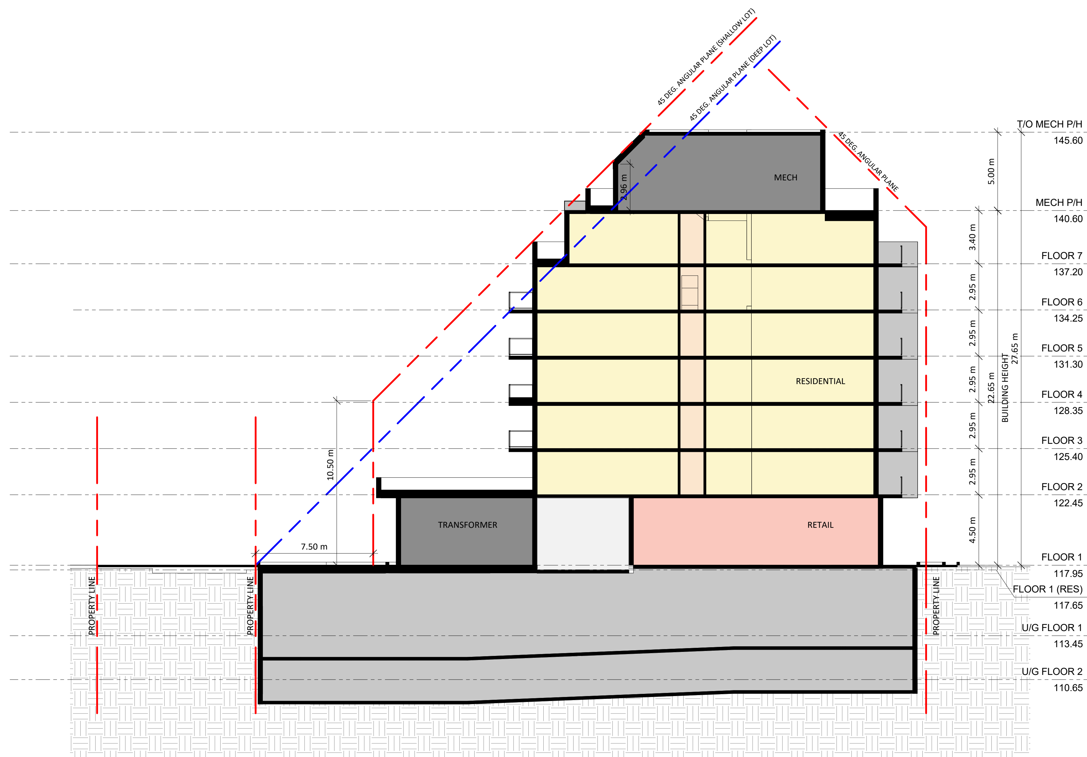
C SECTION C 1 : 150
