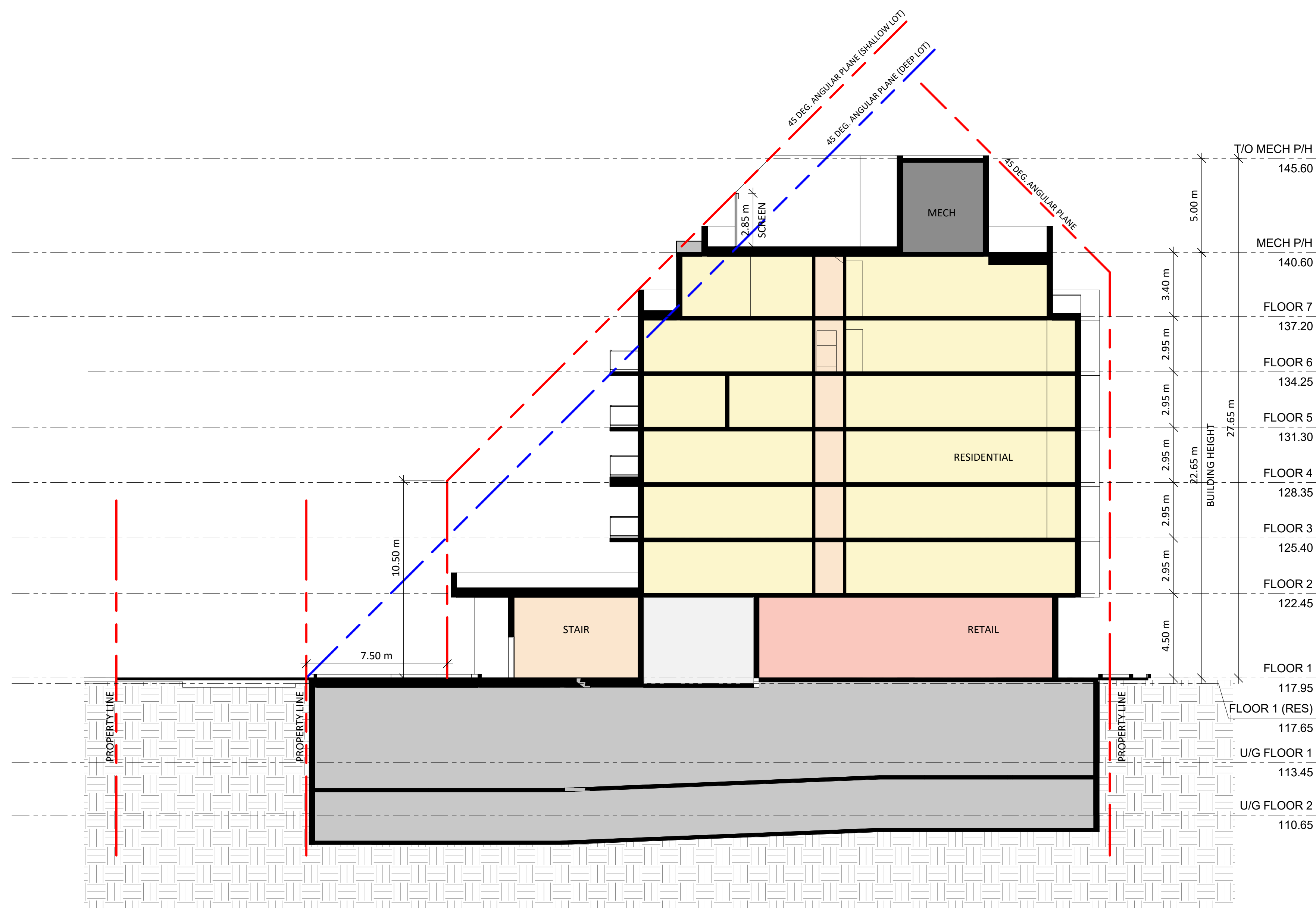
B SECTION B 1 : 150
