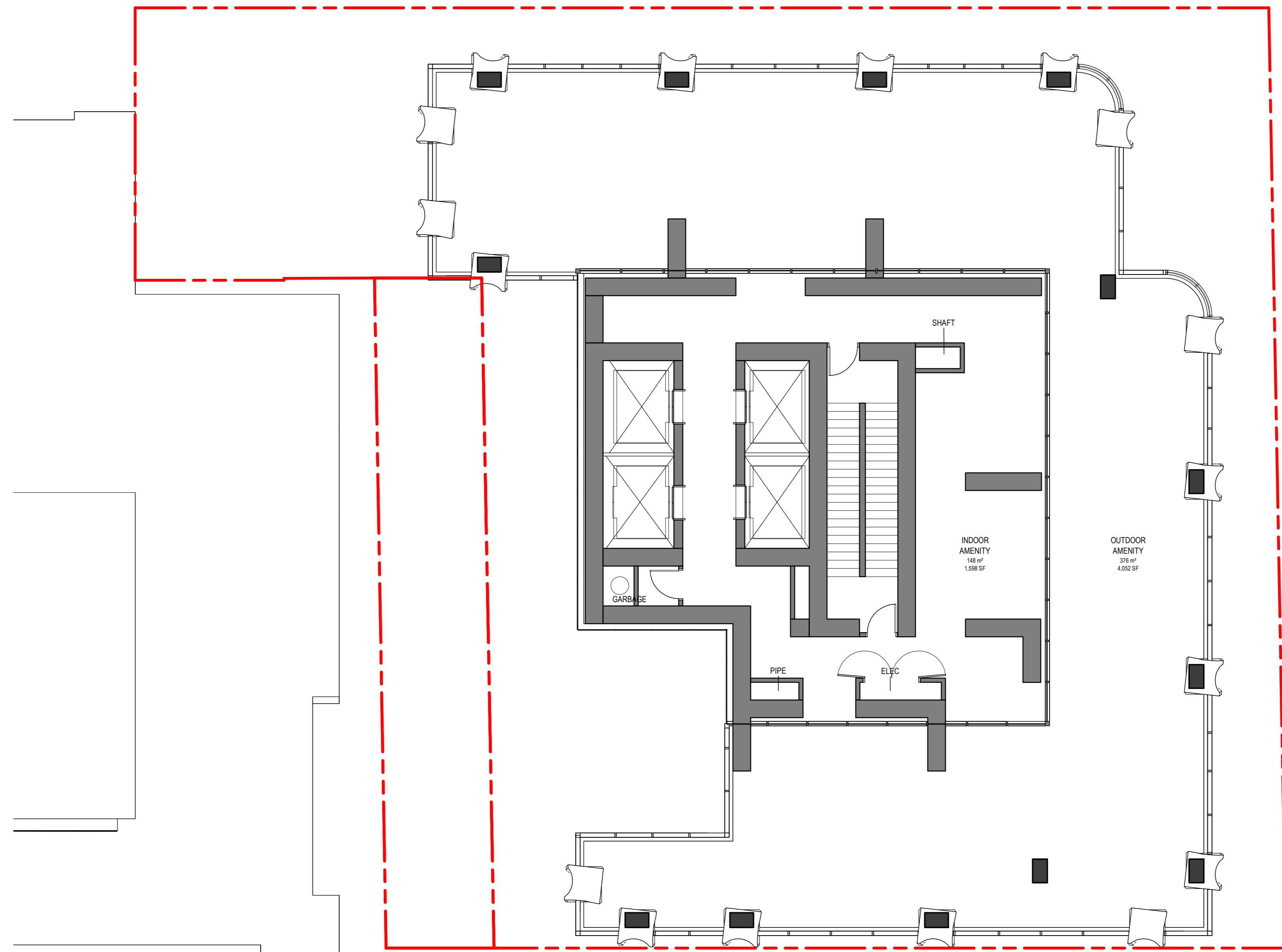
1 L31, L60 TYP AMENITY DP2.4 SCALE: 1:100
