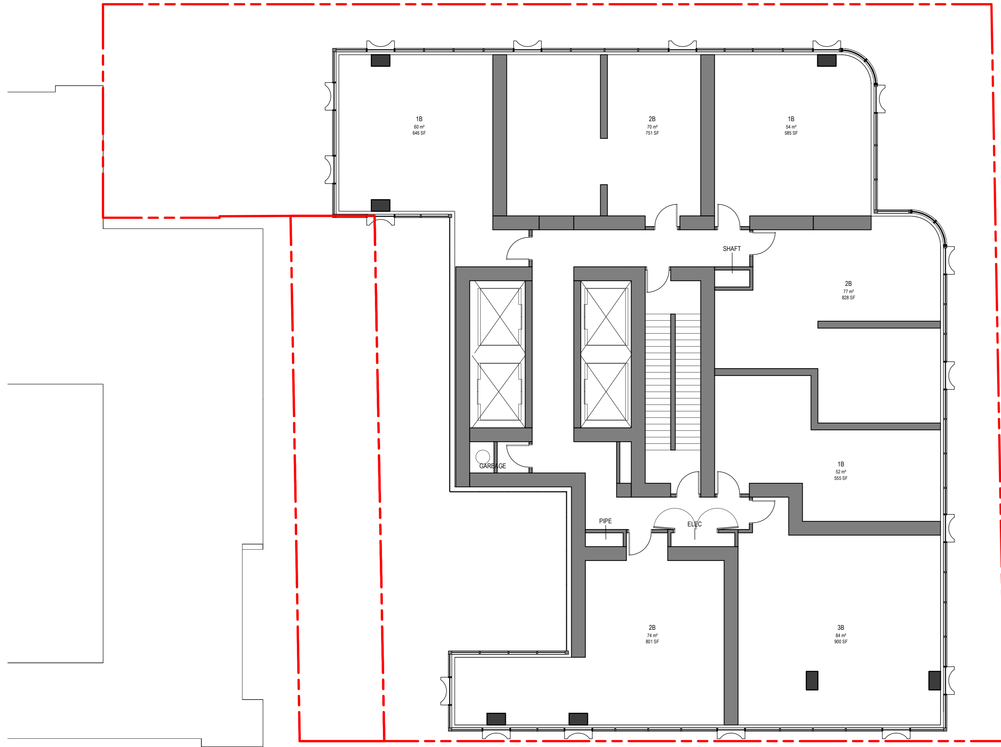
4 TYP TOWER PH DP2.3 SCALE: 1:100
