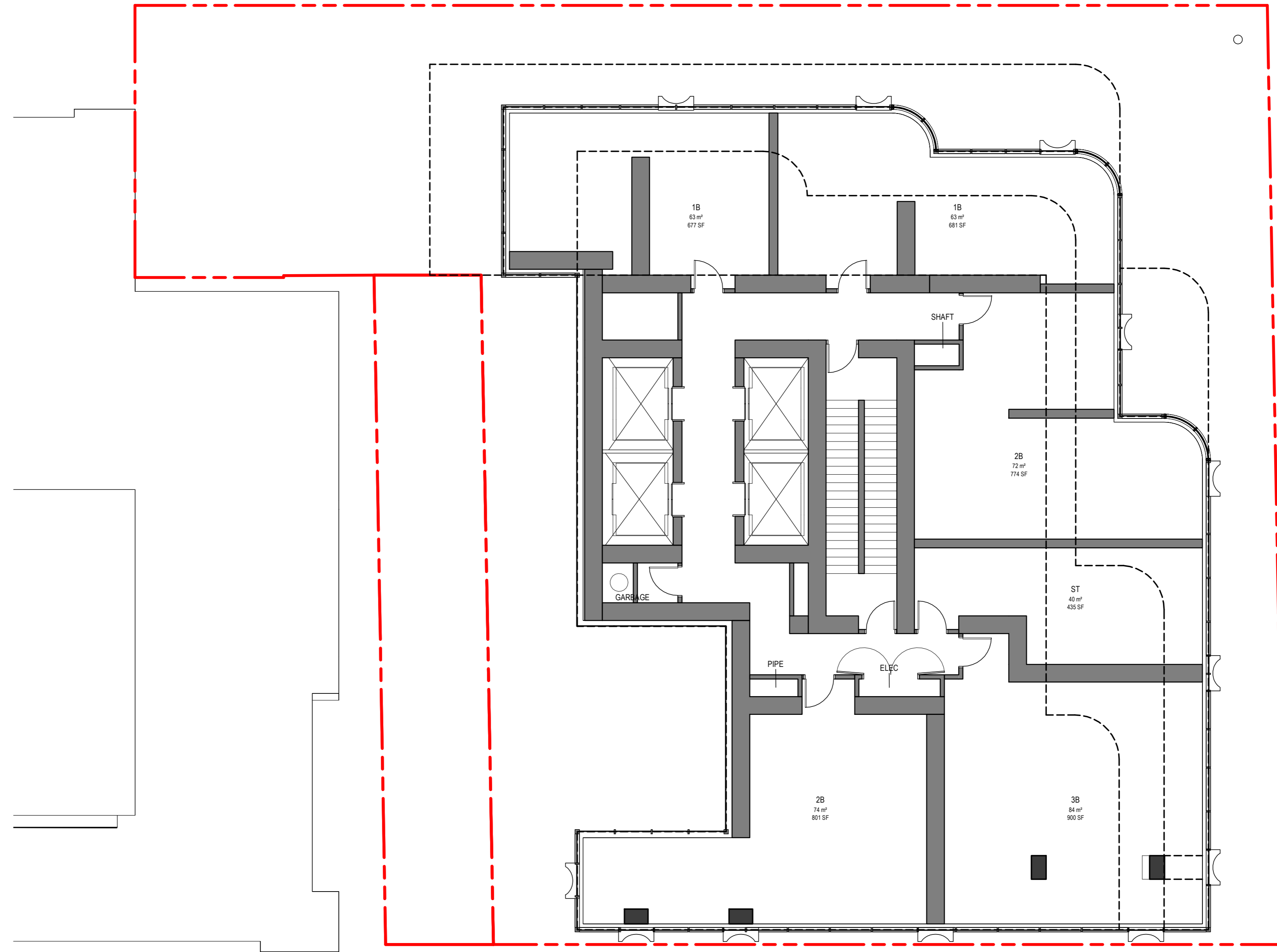
3 L7-8 DP2.3 SCALE: 1:100
