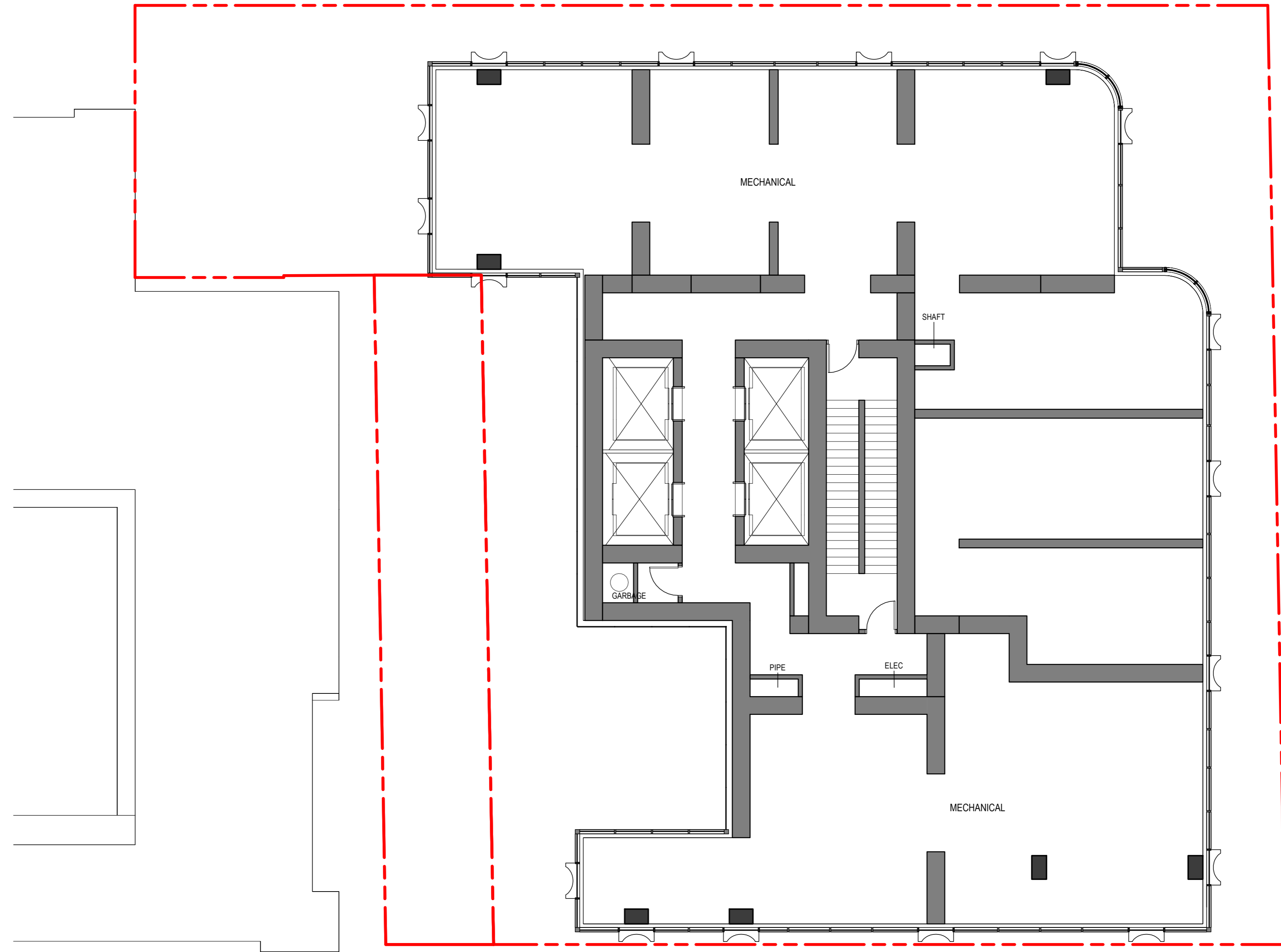
2 L33-34, L62-63 TYP MECH DP2.4 SCALE: 1:100
