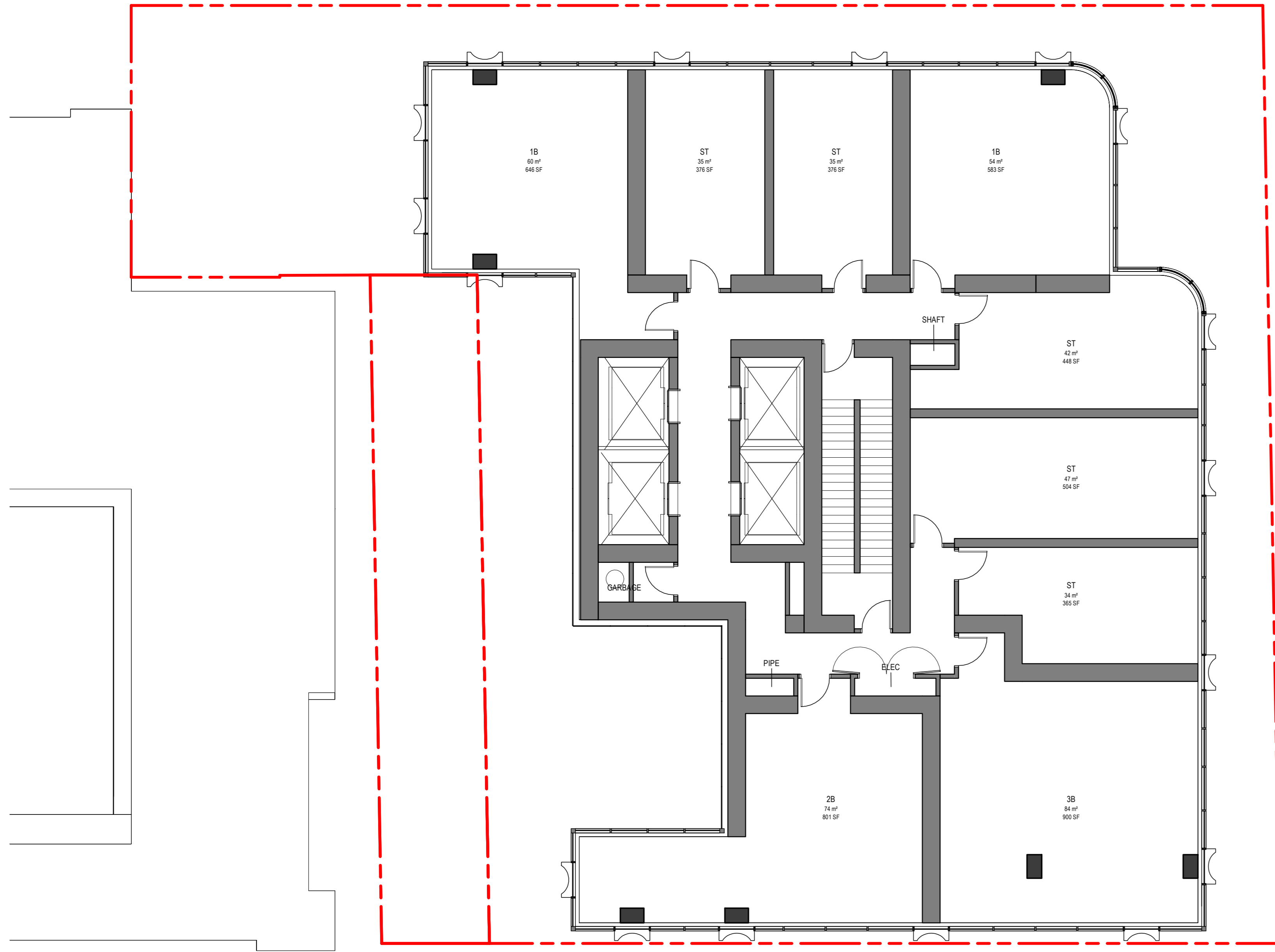
1 TYP TOWER DP2.3 SCALE: 1:100
