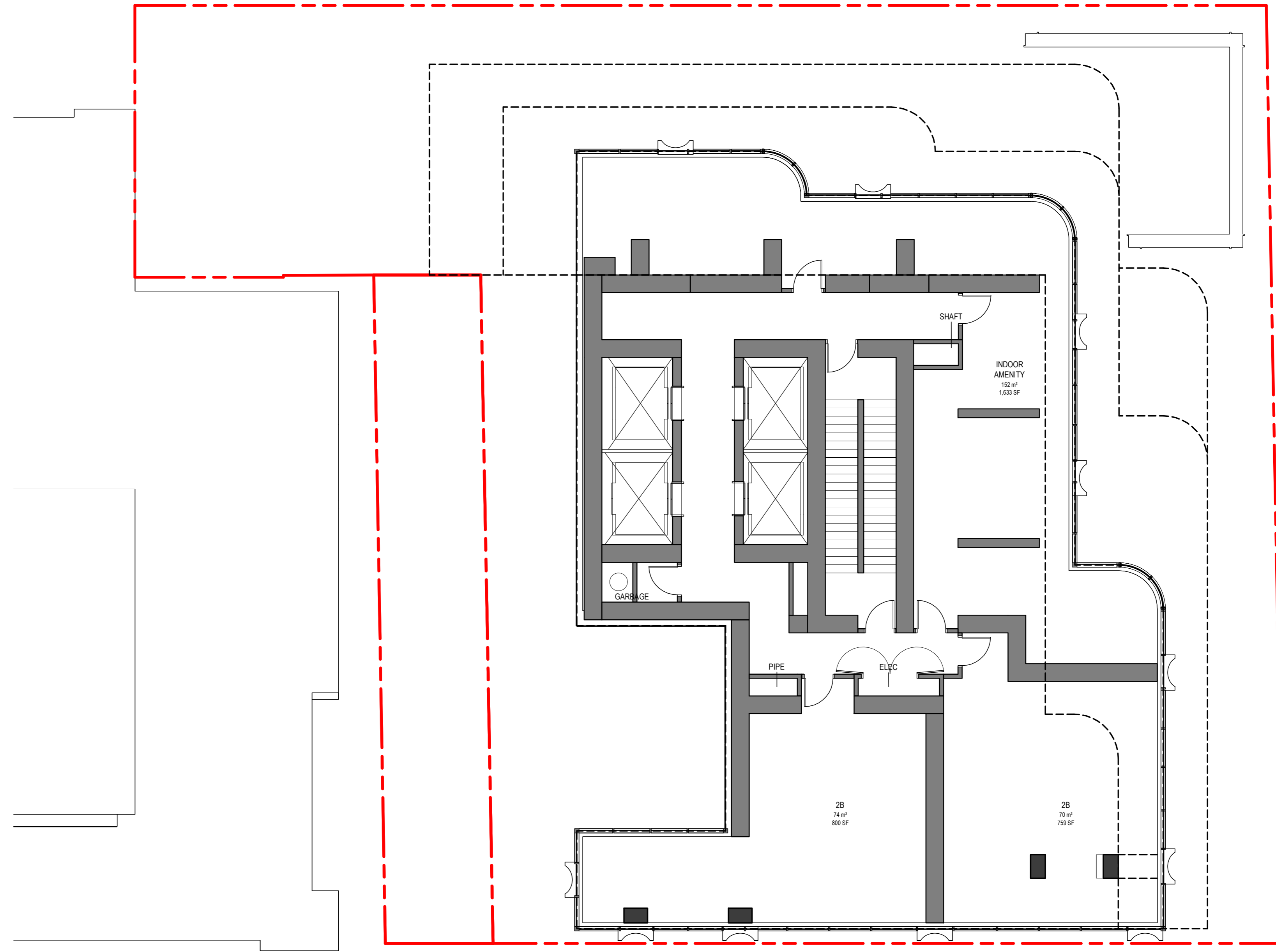
2 L5-6 DP2.3 SCALE: 1:100
