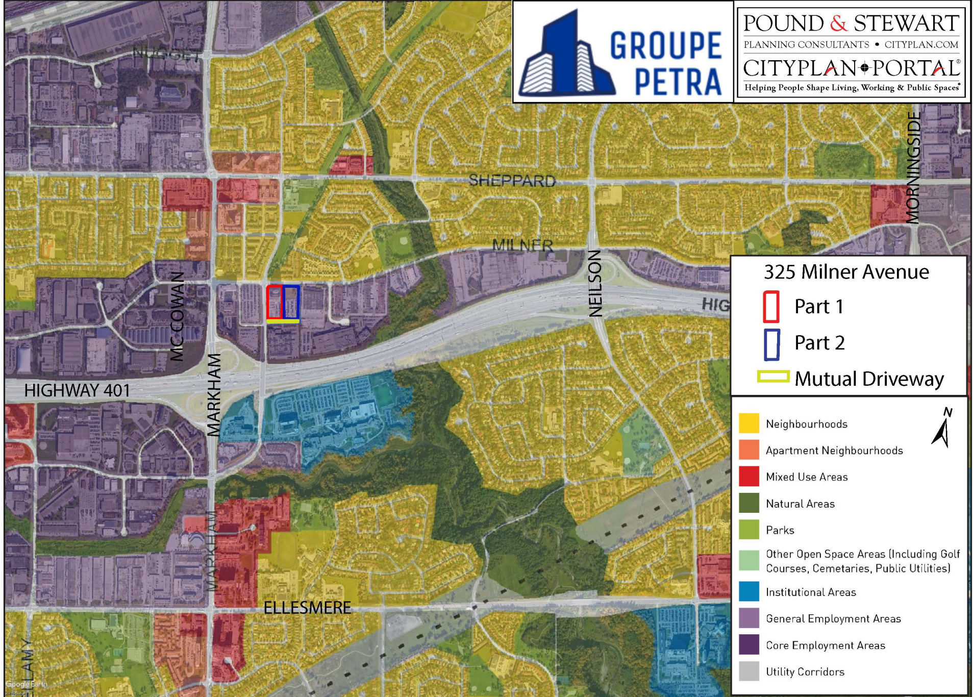
Figure1_TOP_MAP22_LandUse_Jan.2024
