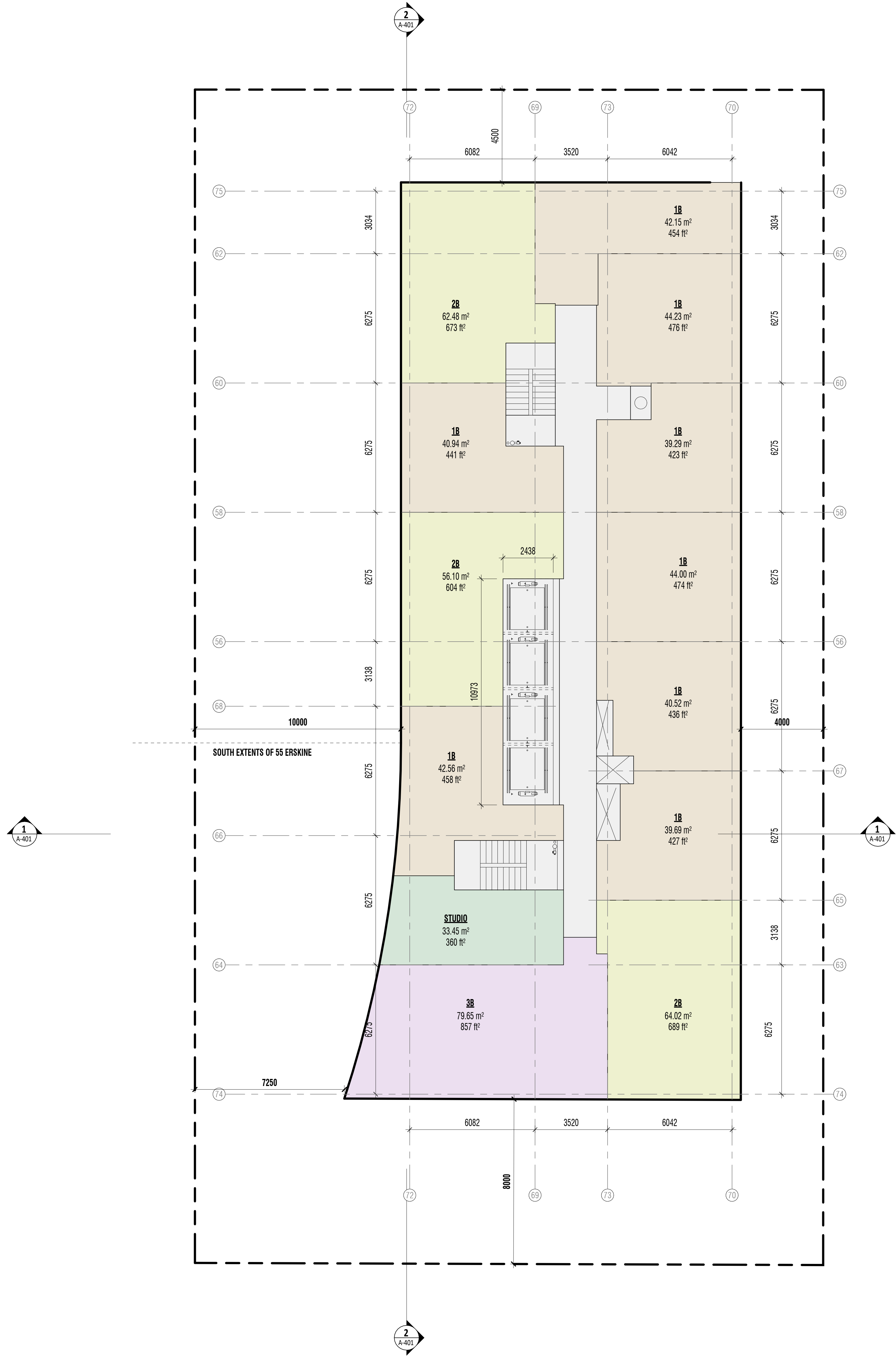
1 LEVEL 12-42 FLOOR PLAN A-301 | A-204 1 : 100
