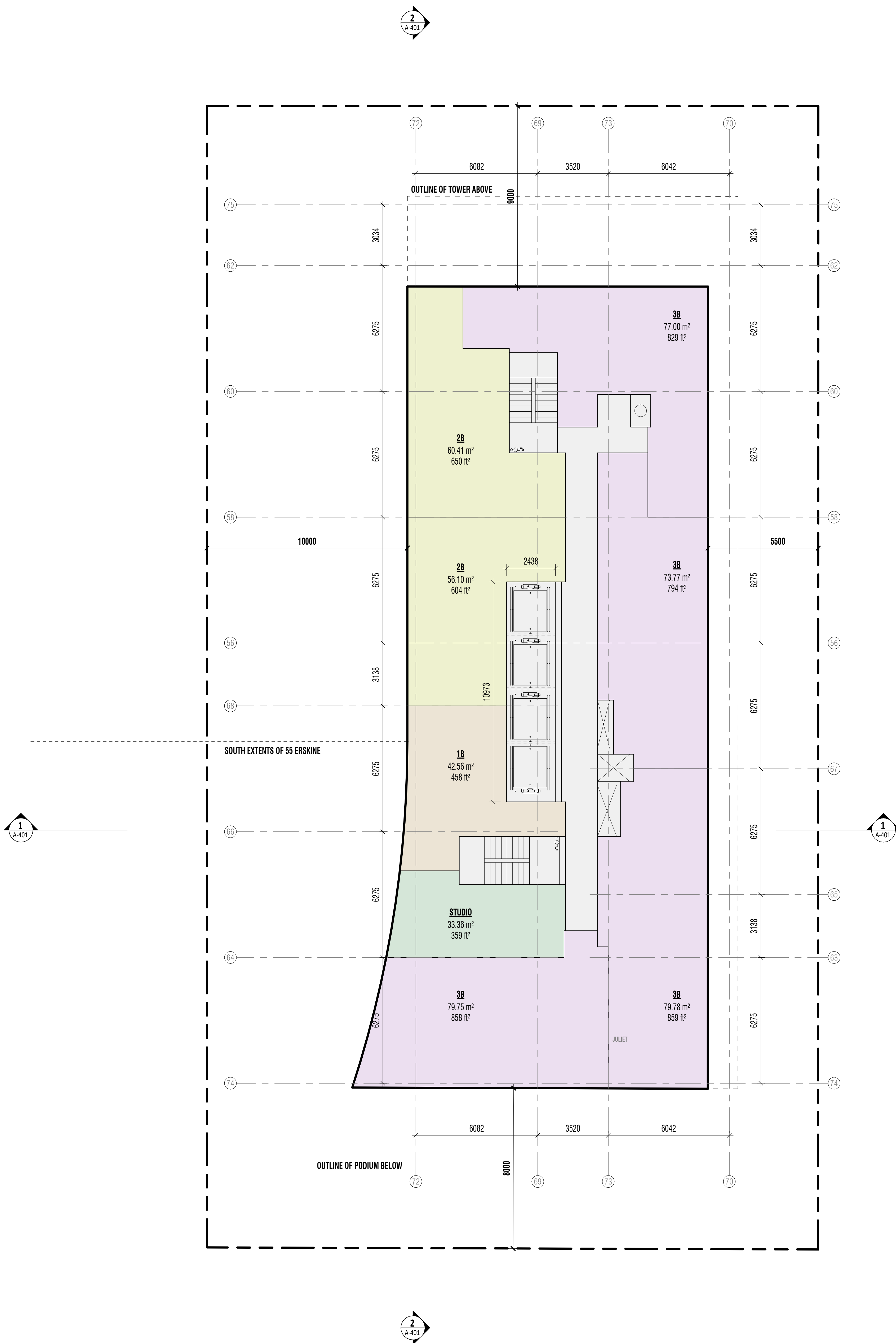
2 LEVEL 7-9 FLOOR PLAN A-301 A-203 1 : 100
