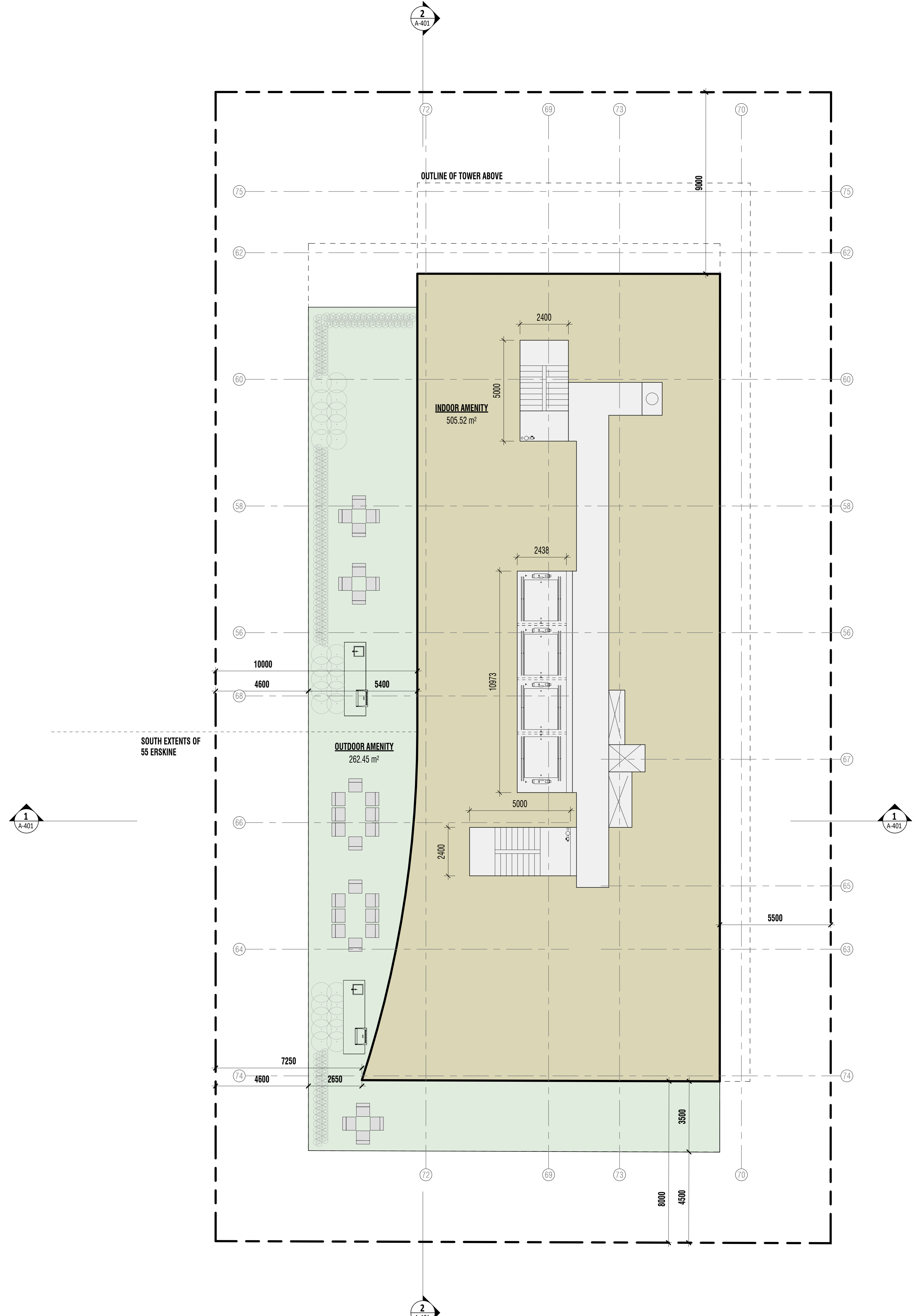
2 LEVEL 6 FLOOR PLAN A-301 A-202b 1 : 100
