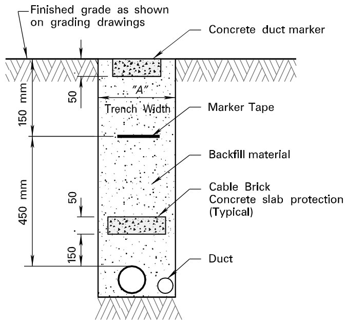
TRENCH ELEVATION
