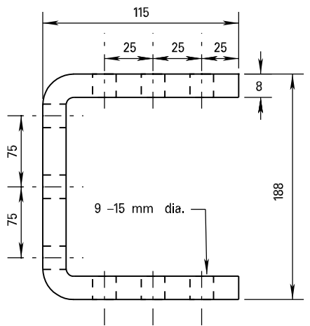
BRACKET 'B'
