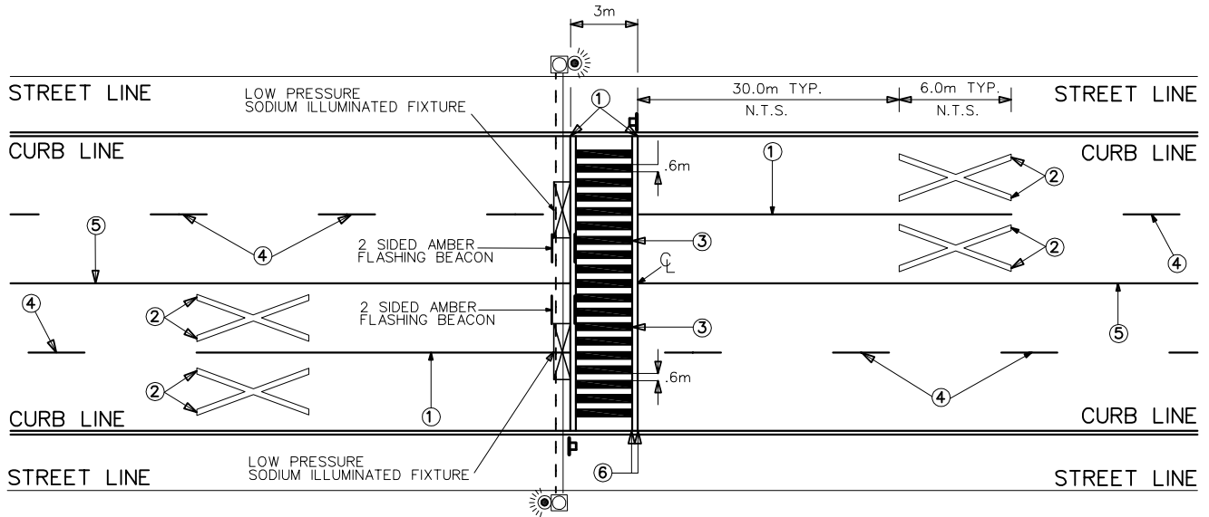
PLAN LAYOUT (N.T.S.)
