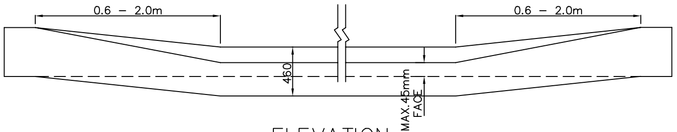
ELEVATION
