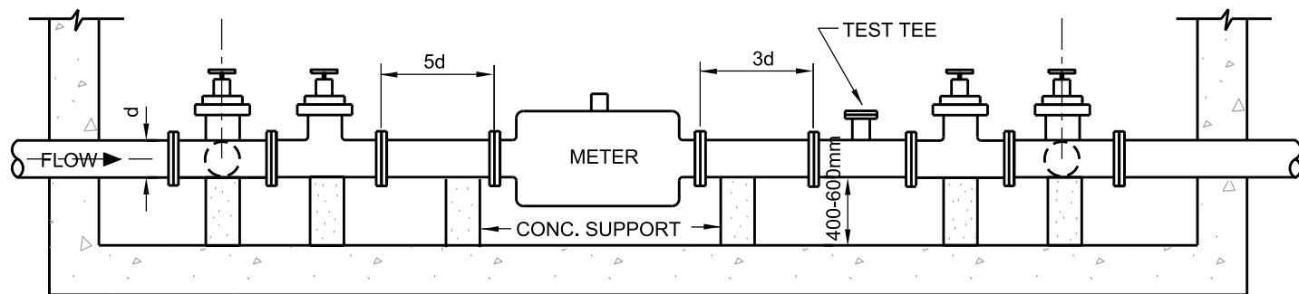
ELEVATION
