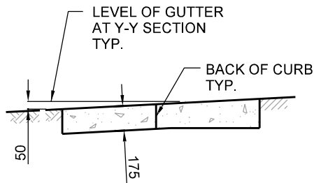
SECTION Y - Y
