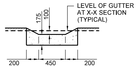
SECTION Y - Y
