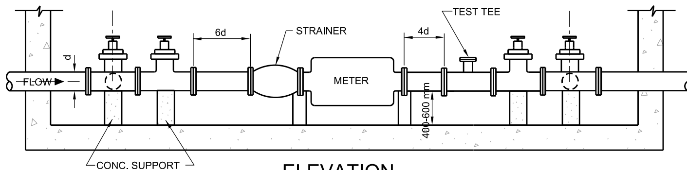
ELEVATION
