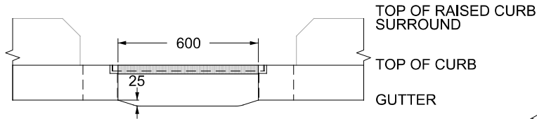
ELEVATION B-B
