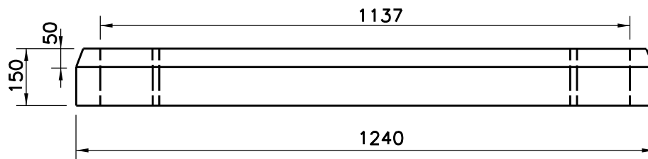
ELEVATION
