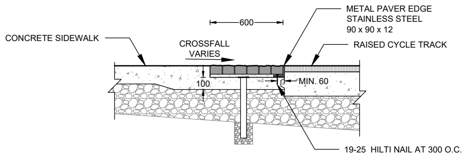
DETAIL 1 - METAL CURB EDGE
