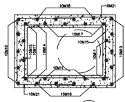
SECTION (D)
