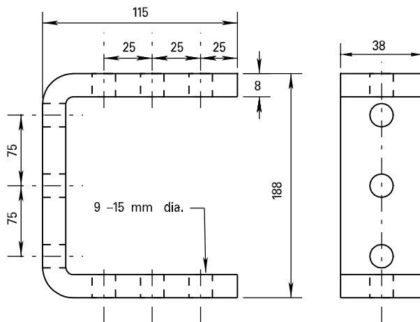
BRACKET 'B'
