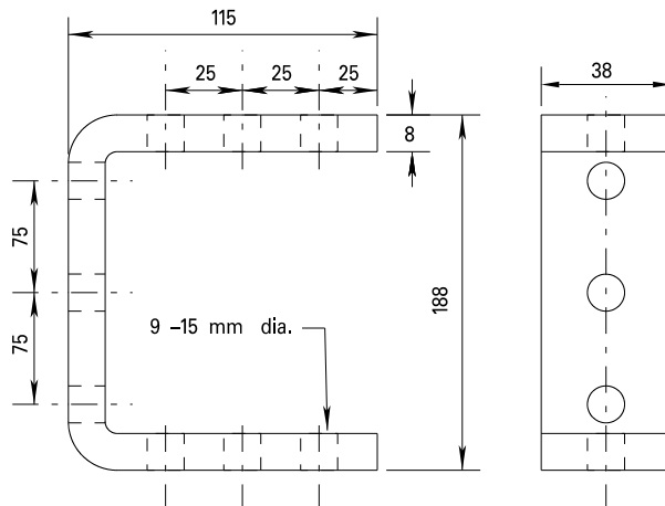
BRACKET 'B'
